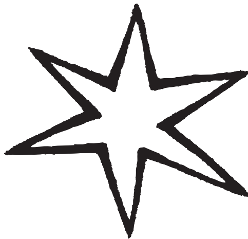
Ruch wybuchowy
